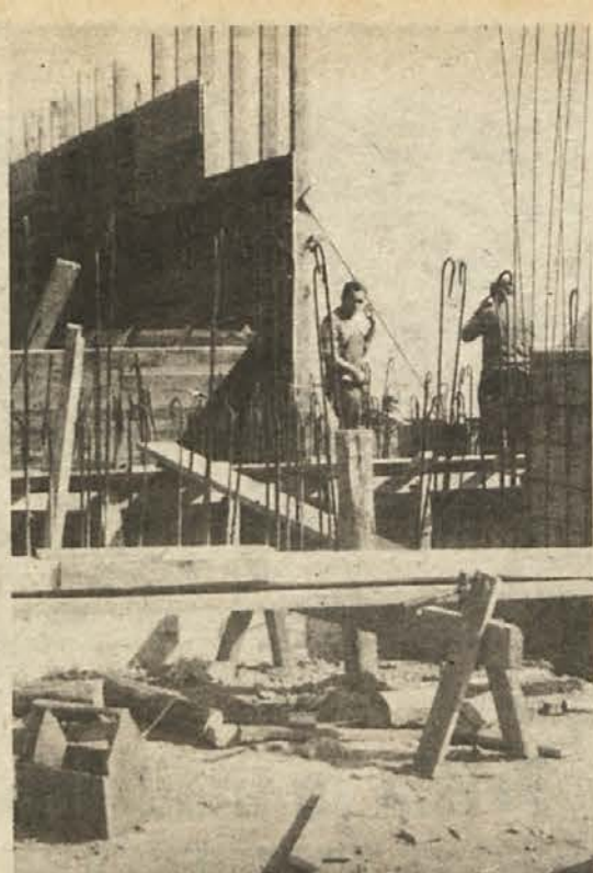
METLIŠKA ČISTILNA NAPRAVA — Ob cesti proti Rosalnicam raste v Metliki centralna čistilna naprava, skozi katero bo spreljana vsa mestna kanalizacija; prečiščene odpadne vode bodo potem tekle v Obrh in naprej v Kolpo. Čistilna naprava bo zgrajena do novega leta. (Foto: Bartelj)
