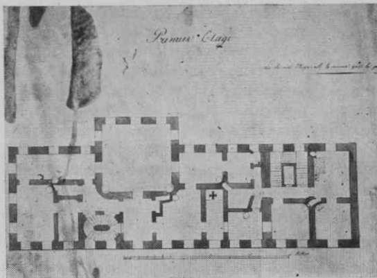
Sl. 12. Načrt Gruberjeve palače iz francoske dobe (1809–1813, DAS)
