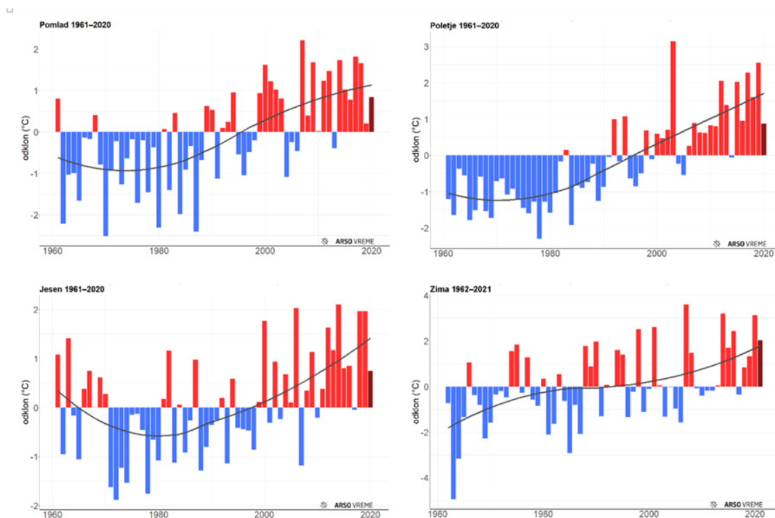
Slika 12-2: Odklon povprečne sezone temperature od povprečja 1981–2010 (modri in rdeči stolpci) in večletno glajeno povprečje (črna krivulja)
