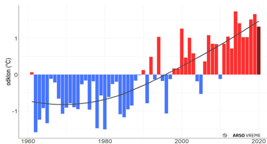
Slika 12-1: Odklon povprečne letne temperature od povprečja 1981–2010 (modri in rdeči stolpci) in večletno glajeno povprečje (črna krivulja)
