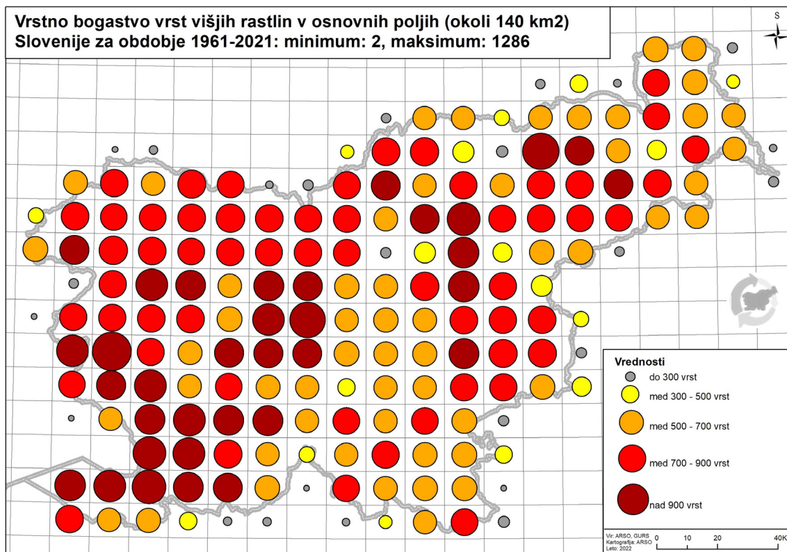
Slika 5-5: Vrsto bogastvo vrst višjih rastlin v osnovnih poljih (okoli 140 km 2 ) Slovenije za obdobje 1961-2021: minimum: 2, maksimum: 1286; . Temnordeča: >900 vrst, svetlordeča: 700-900, oranžna: 500-700, rumena: 300-500, siva: do 300 vrst
