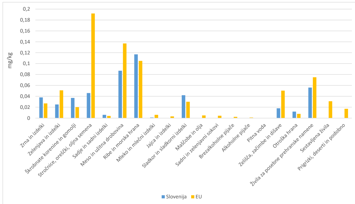
Slika 20-8: Najvišje povprečne koncentracije kadmija (Cd) so bile v Sloveniji zaznane v ribah in morski hrani, v EU pa tudi v stročnicah, oreščkih in oljnih semenih
