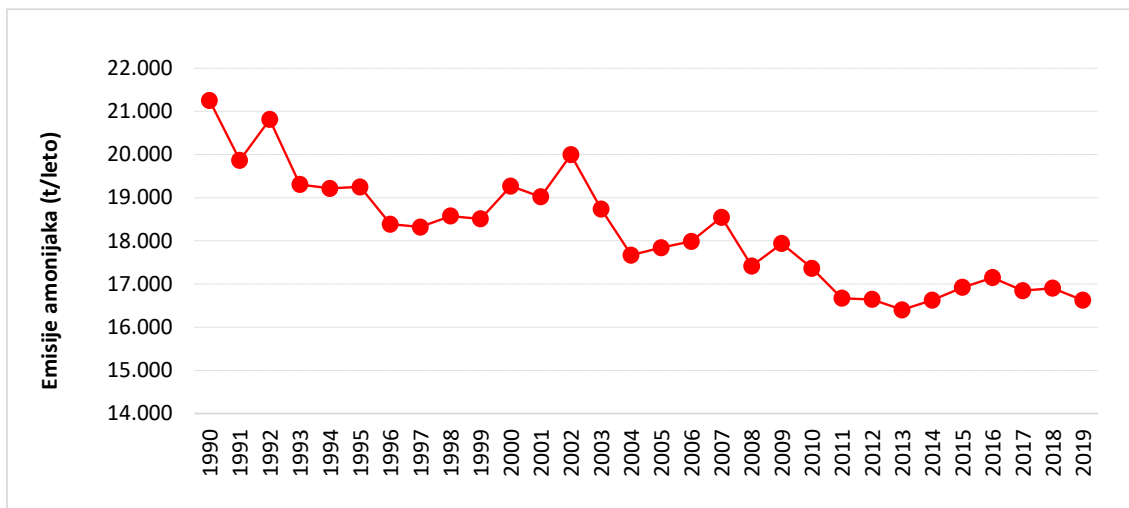
Slika 17-12: Gibanje letnih izpustov amonijaka v kmetijstvu. V obdobju 1990–2019 so se izpusti zmanjšali za 21,8 %. Kmetijstvo na področju izpustov sledi cilju, ki ga za leto 2020 določa Direktiva o zmanjšanju nacionalnih emisij za nekatera onesnaževala zraka (Ur. l. EU, 2016).
