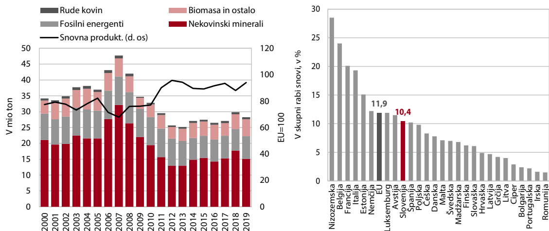
Slika 15-2: Domača poraba snovi in relativna snovna produktivnost, Slovenija (levo), ter stopnja porabe predelanih snovi, leto 2019 (desno)
