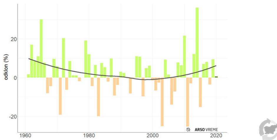
Slika 12-7: Odklon povprečne sezone višine padavin od povprečja 1981–2010 (zeleni in rjavi stolpci) in večletno glajeno povprečje (črna krivulja)
