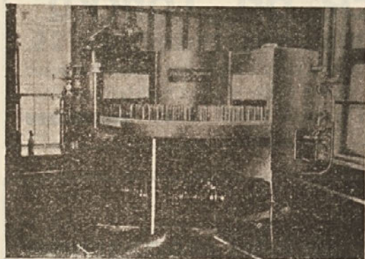
Najmodernejši stroj za pranje steklenic „Cerevisia Injektor“, edini v Jugoslaviji
