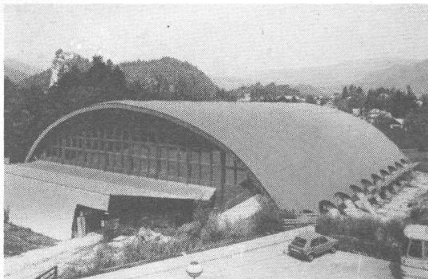
Športna dvorana na Bledu je zgrajena z uporabo lepljenih nosilcev v izvedbi Hoje
