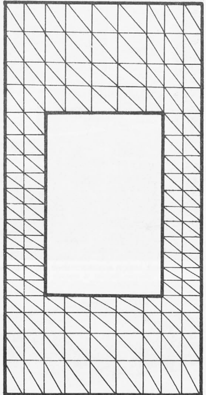
Slika 4: Dvodimenzionalna mreža končnih elementov okvira stiskalnice
