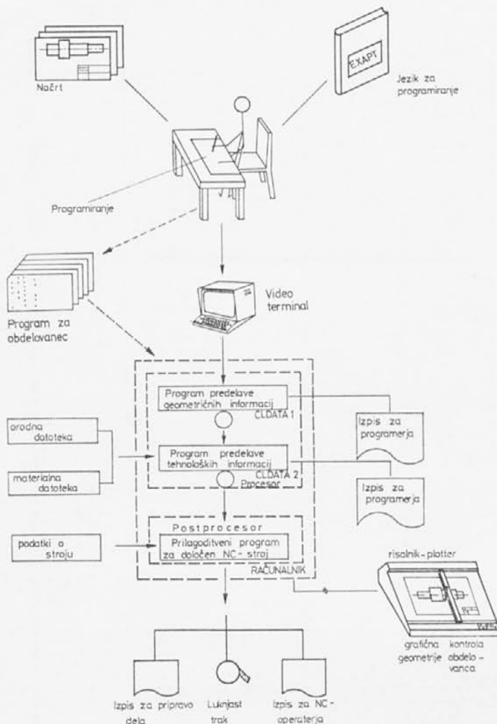
Slika 2: Potek obdelave programa za obdelovance po EXAPT-programskem paketu
