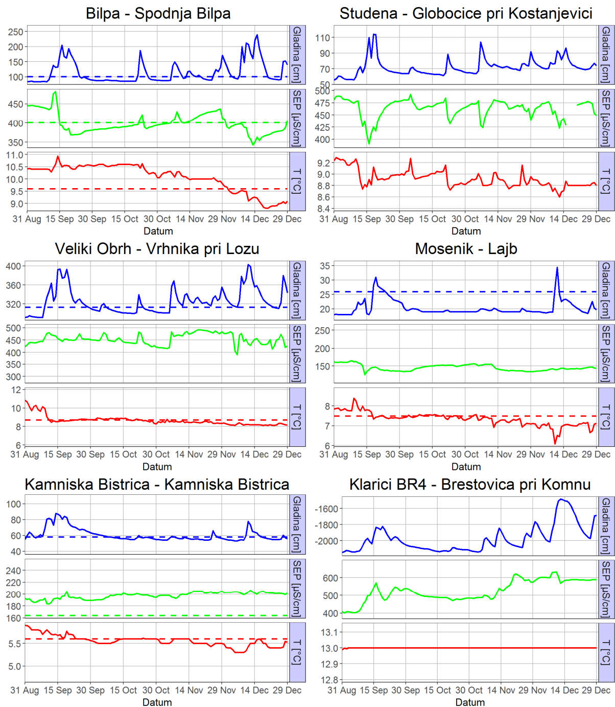
Slika 3. Nihanje vodne gladine (modro), temperature (rdeče) in specifične električne prevodnosti (zeleno) na izbranih merilnih mestih izvirov in podzemne vode v Klariči na območju Krasa med septembrom in decembrom 2017
