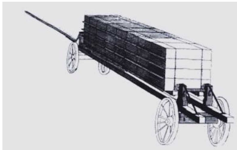
Voz za prevažanje čebelnih panjev (Janša, 1775) – Crane (1999, str. 350)
