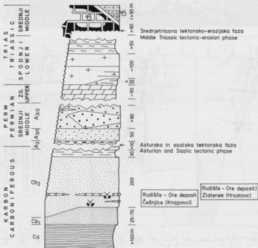
Sl. 3. Geološki stolpec območij Češnjice-Zlatenec
