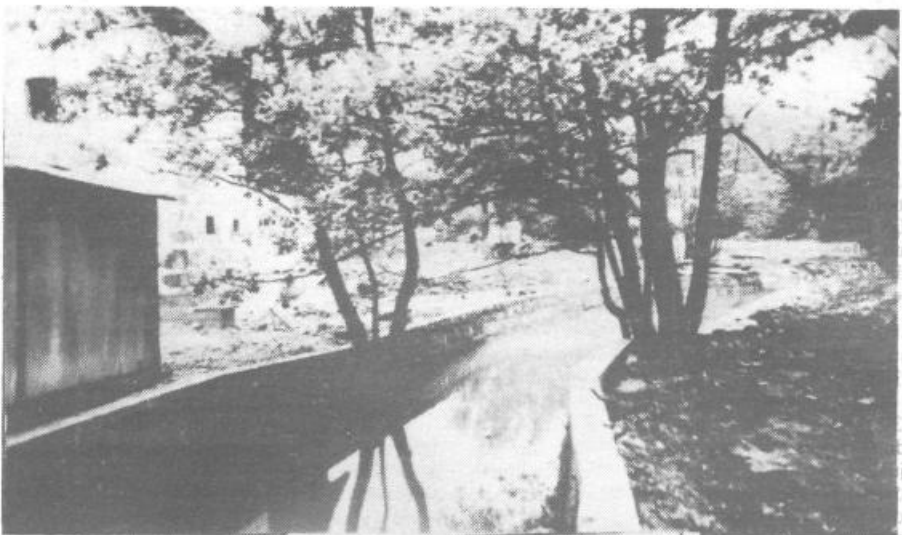
V okviru urejevalnih del Trubarjevega spominskega gaja je OVS Ljubljana-Sava uredila del struge v Rašici ter obnovila jezovno napravo pri Trubarjevem mlinu. Zgradila je tudi 28 m dolg obrežni zid, odpeljala 222 kubičnih metrov lomljenca in na celotnem odseku posekala grmovje in dreve.
