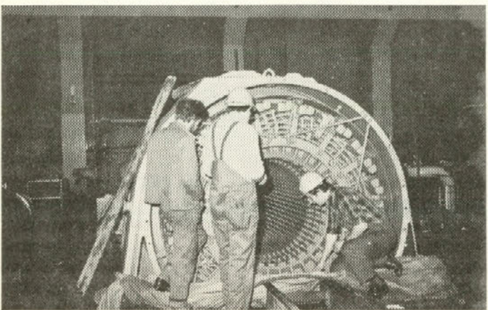
Z letošnjega rednega letnega remonta blokov I. faze TEŠ (2 x 30 MW) – ZGORAJ: Pri reviziji turbin je bilo treba natančno pregledati tudi vsako lopatico nizkotlačnega dela rotorjev. SPODAJ: Kontrola navitja statorja pri enem od generatorjev
