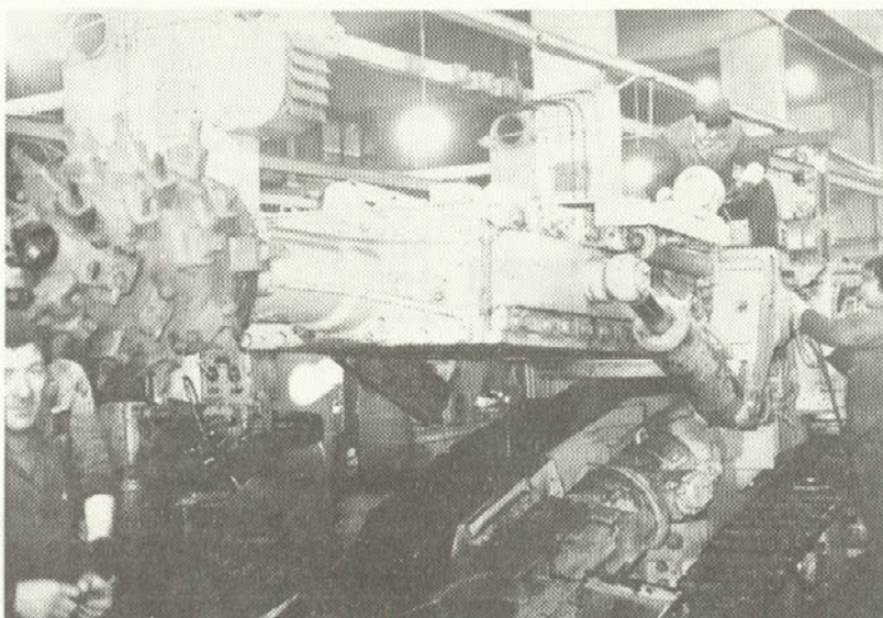
Tik pred koncem izpopolnjevanja stroja PK - 9R za izdelavo jamskih prog v našem rudniku
