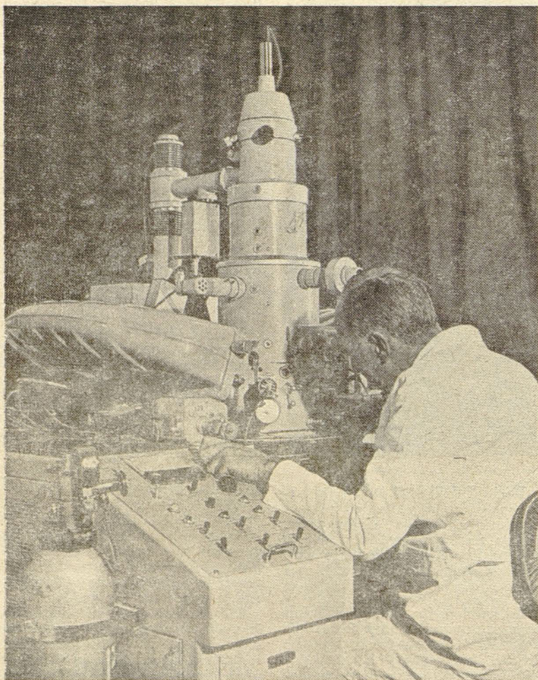
Elektronski mikroanalizator v metalurškem inštitutu Ljubljana
