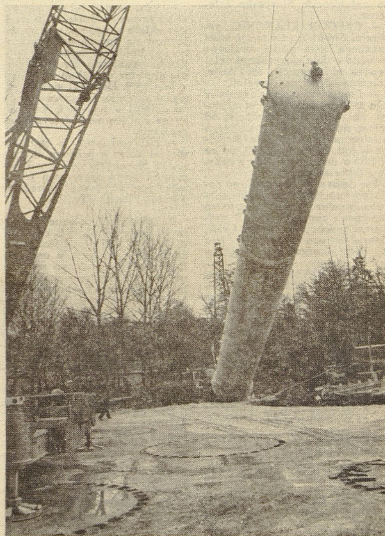
Kot raketa, se počasi dviga in približuje prvi rezervoar montažnemu mestu (krog ob vznožju slike)
