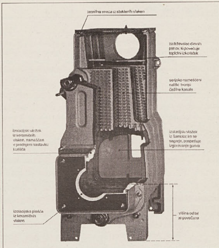
Litoželezni kotel na tekoče ali plinasto gorivo
