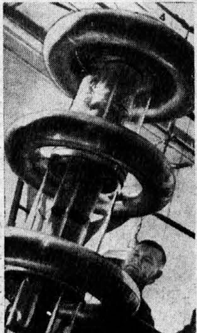
Na sliki vidimo tri dele ogromne röntgenske cevi, ki jo je izdelala ameriška tvrdka General Electric Company za poldrugi milijon voltov napetosti.
