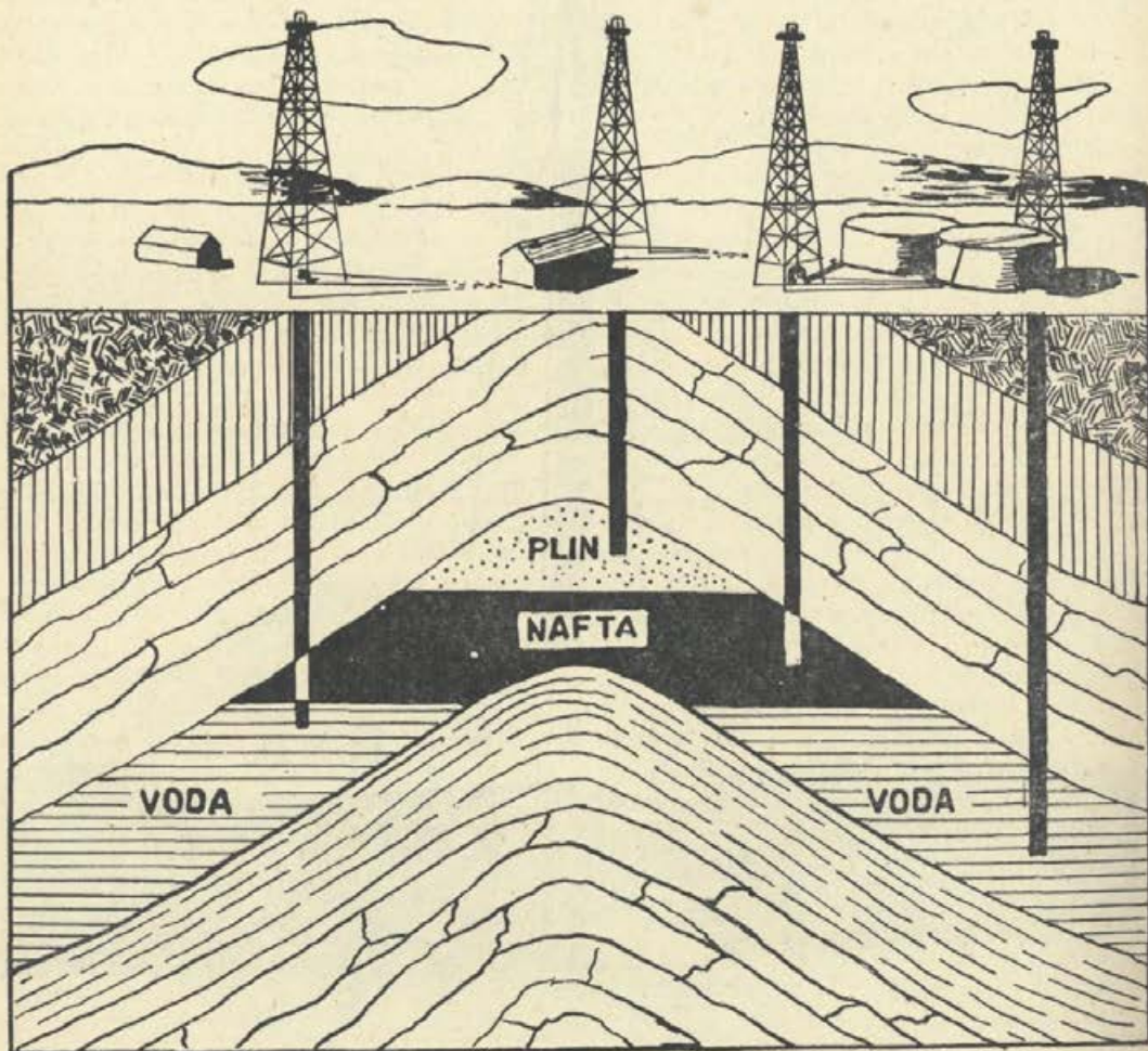
Prerez skozi naftno polje. Stolpi za vrtanje so najbolj značilna zunanja podoba naftnih področij.
