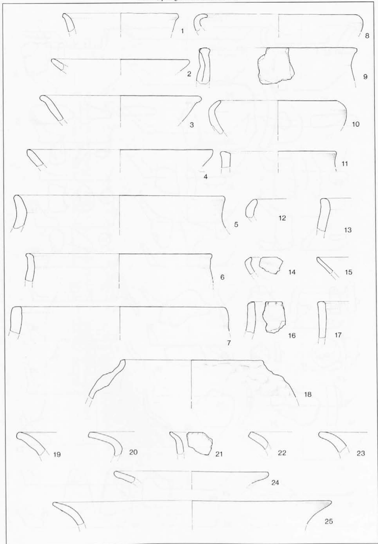
T. 2: Kostel. Sonda 1. Vse glina. M. = 1:3.
