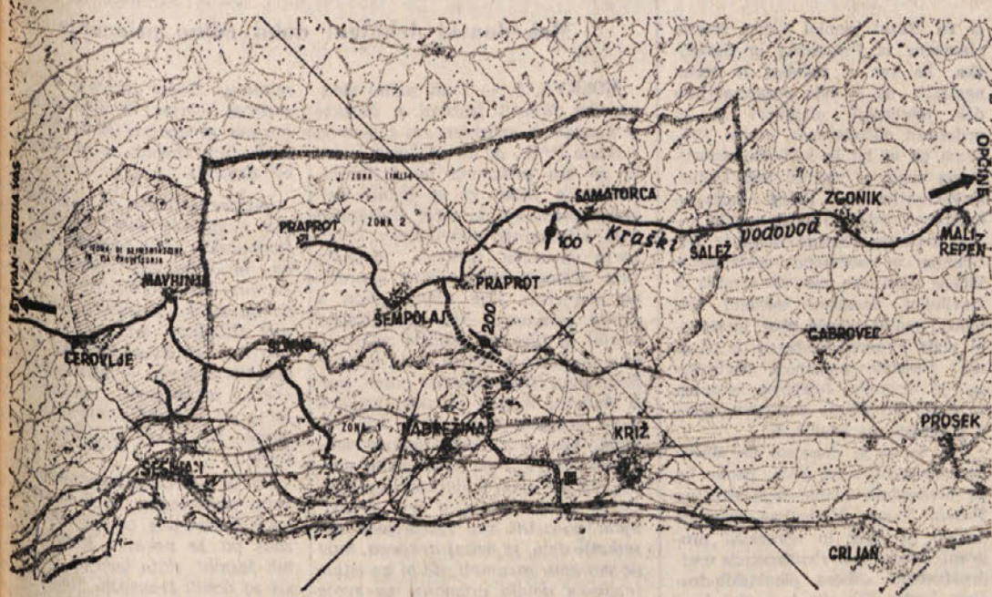
Omrežje Kraskega vodovoda
