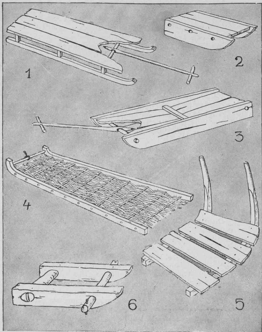
Sl. 2. Razne sani: 1. miške — sani za prevoz rude (Dražgoše); 2. marjaše — sani za sankanje (Sv. Ana nad Tržičem); 3. űačuje — sani za razvažanje gnoja po strmih njivah (Jezersko); 4. gratula — sani za razvažanje gnoja (Črna); 5. plakuže — sani za kamenje (Martinj vrh); 6. smake — sani za vlačenje lesa (Štiška vas pod Krvavcem)
