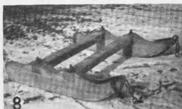
Sl. 1. Vprežne sani za gnoj (Lom); 2. vprežne sani s templanci (Četena ravan); 3.—5. vprežne sani za les (Koroška Bela, Četena ravan in Kupljenik); 6. podaljšane sani (Lom); 7. vožnja hlodov na saneh s podloženim skokom (Bohinj); 8. skok, sani za podkladanje pod hlode (Stara Fužina)
