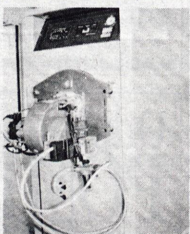
Peč Elkoterm za pripravo sanitarne vode poleg centralnega ogrevanja stanovanjskih prostorov je visoka 105, široka 55 in globoka 70 centimetrov.
