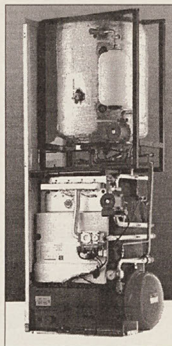
Kotel z akumulacijskim bojlerjem 85l (VARIANTA B)
