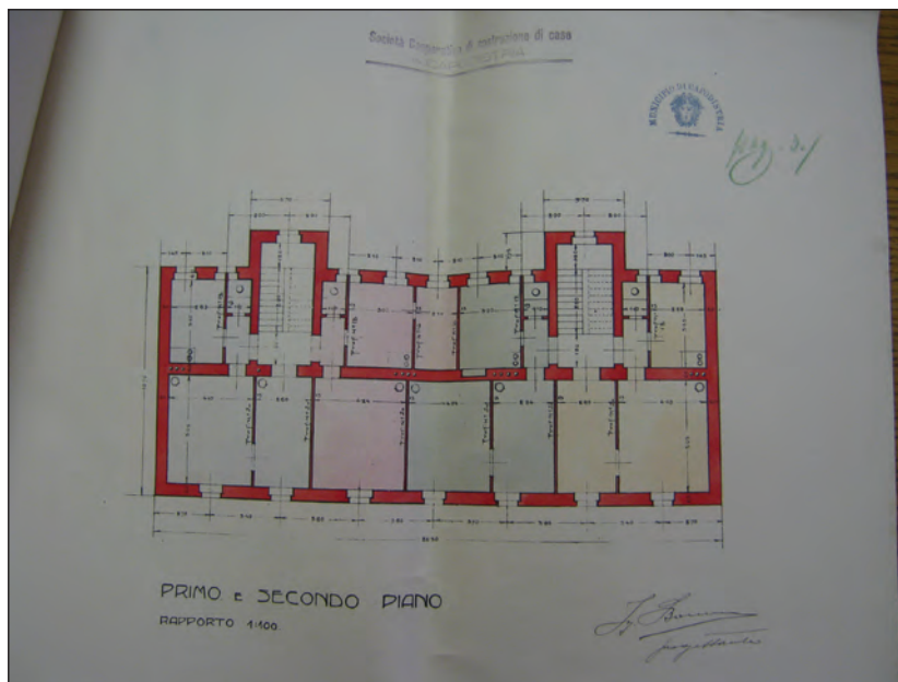
Slika 6: Tloris prvega in drugega nadstropja stavbe »casa operai« (SI PAK-22, 3, 8) (foto: N. Čebtron Lipovec)
