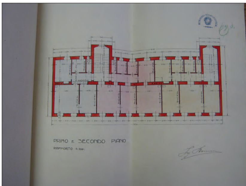
Slika 7: Tloris prvega in drugega nadstropja stavbe »casa impiegati« (SI PAK-22, 3, 8) (foto: N. Čebtron Lipovec)
