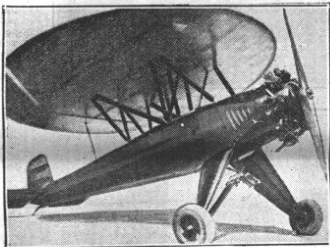
CLOVEK POSNEMA NARAVO. V Ameriki so zgradili letalo v obliki kobilice
