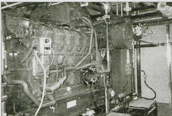
Napravo poganja plinski motor, ki poganja generator, ta pa soproizvaja električno in toplotno energijo.
