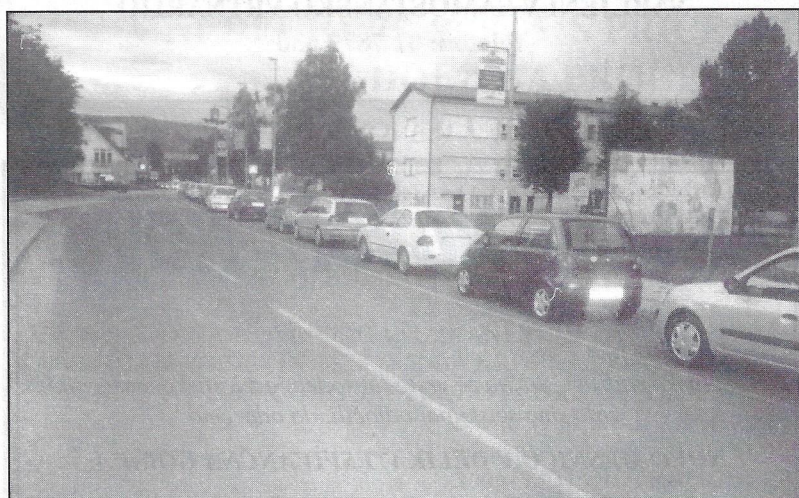
Največji delež antropogenih izpustov CO 2 povzroča promet.
