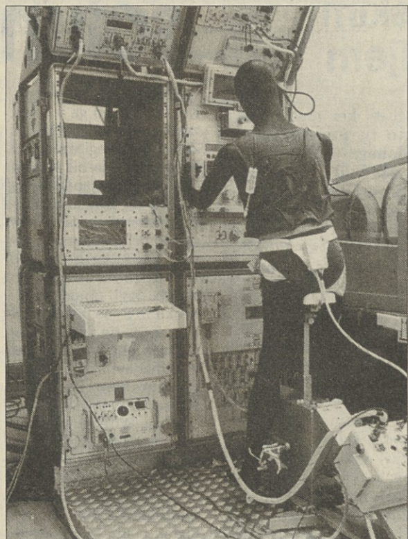
Neenavaden medicinsko-psihološki laboratorij: antropološki sistem z 19 moduli za preizkuse
