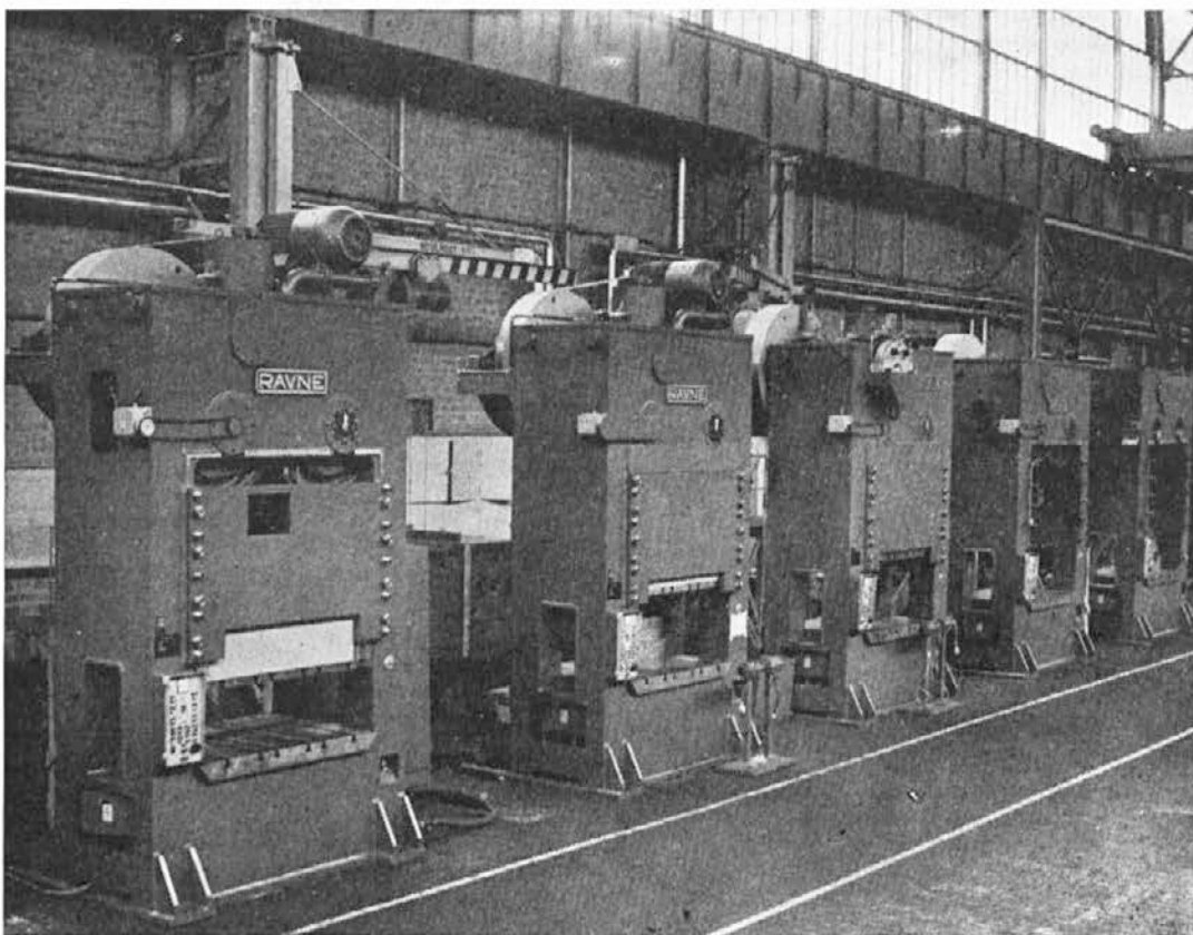
Serijske stiskalnice 4000 KN, dobavljene v SSSR v juniju 1976
