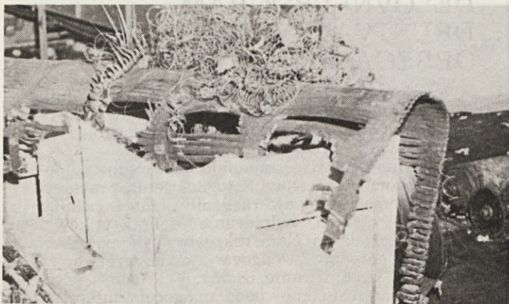
Na stroju Hergeth je pred trgalnim valjem zgorel dovajalni letvasti pas iz plastike. Od plastičnih cevi vidimo na fotografiji samo spiralasto ogrodje cevi.
