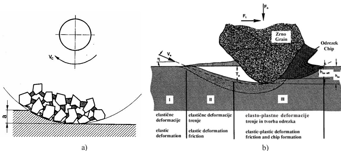
Sl. 1. Makro in mikro načelo brušenja ([5] in [6])
