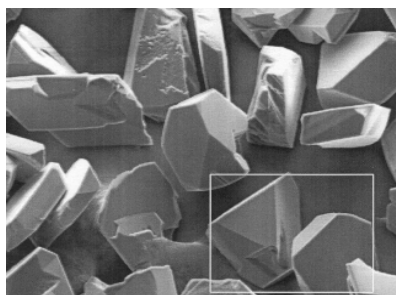
Sl. 2. Mikrostruktura KBN [1] Fig. 2. CBN microstructure [1]
