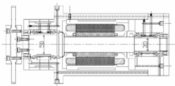
Sl. 9. Zelo hitro vreteno Fig. 9. High speed spindle unit
