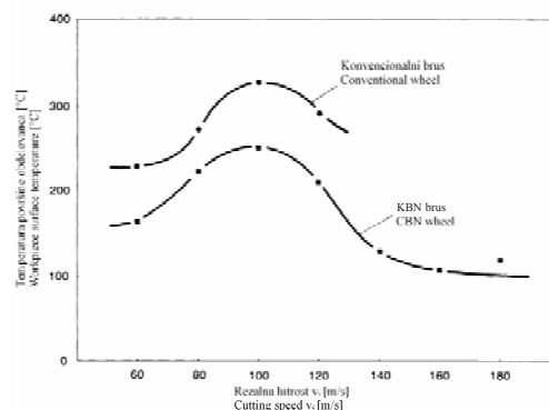
Sl. 6. Porazdelitev temperature obdelovanca [20]
