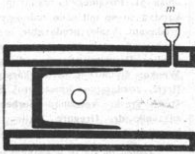
Sl. 7. Ležeči valj v podolžnem prerezu, ki se sčasoma na spodnji strani obrabi; m maznica.
