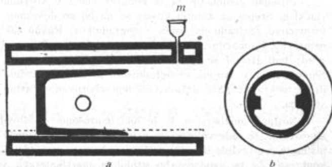
Sl. 8. Ležeči valj, obrabljen na spodnji strani. Temeljito popravilo je nujno potrebno; a v podolžnem prerezu, b v poprečnem prerezu, m maznica.
