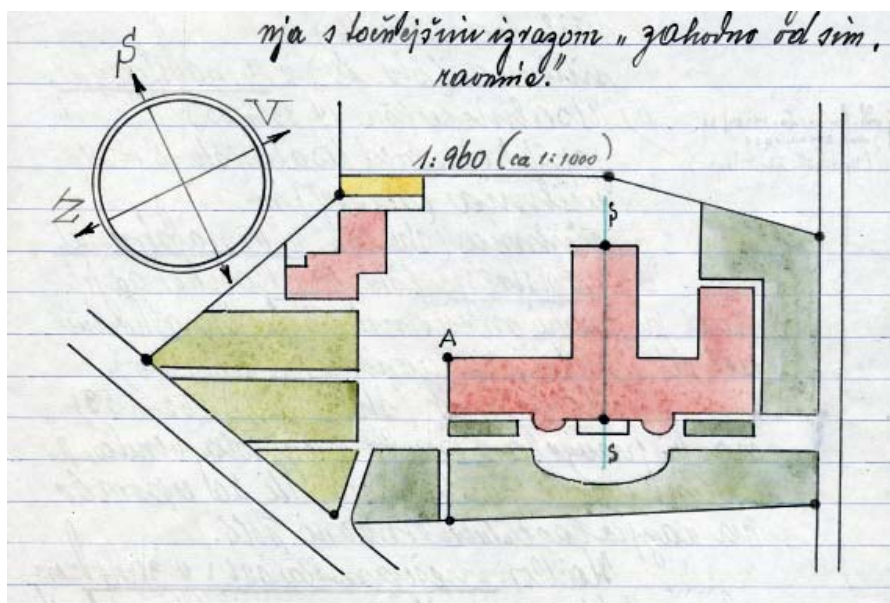
Situacijska skica umestitve novega šolskega poslopja v prostor in predlagana delitev prostorov med meščansko šolo (levo od glavnega vhoda) ter osnovno šolo (desno od glavnega vhoda).
