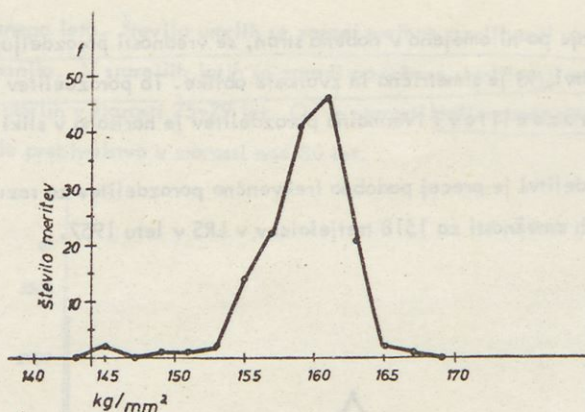
Slika 7.7 Frekvenčna porazdelitev o trdnosti za patentirano 5 mm jeseniško žico v \text{kg/mm}^2 . (Po podatkih Zavoda za raziskavo materiala in konstrukcij SRS)
