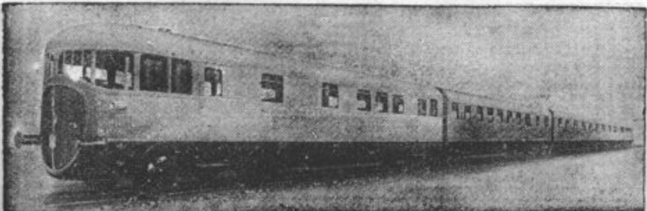
Fiatova tvornica v Turinu je zgradila motorni vlak, ki je dosegel povprečno brzino 160 km na uro. Za pogon služita dva Dieslova motorja po 400 k. s. Montirana sta eden na sprednjem, drugi pa na zadnjem koncu vlaka
