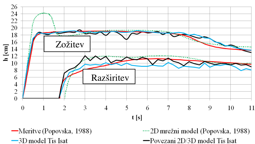
Slika 51: Simulirana in merjena globina v točki zožitve in razširitve kanala
