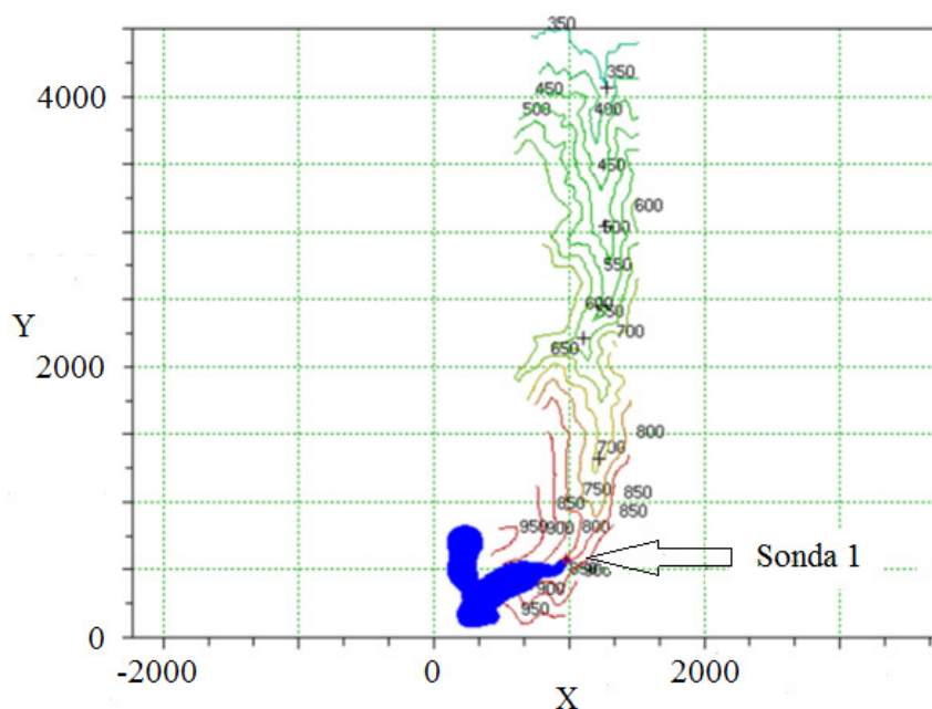
Slika 83: Tlorisni prikaz toka vode 27 s po porušitvi pregrade ( d = 2,5 m; bvis = 0,014 )
