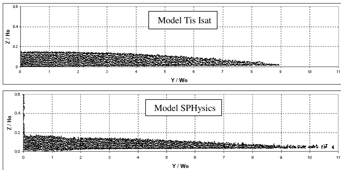
Slika 16: Primerjava napredovanja čela vala 0,3 s po porušitvi pregrade; H_o/W_o = 2 , število delcev je 50 x 100 (Petkovšek in sod., 2010 a)
