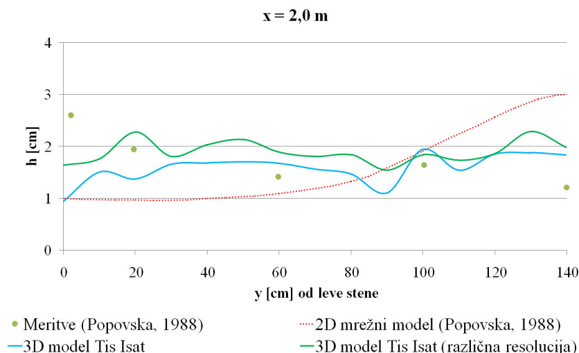
Slika 54: Prečni profil (od leve stene do sredine kanala) na razdalji 2 m od razširitve; t = 5 s.
