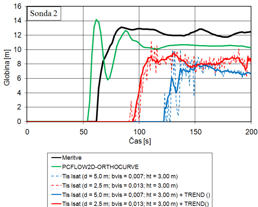
Slika 104: Nihanje gladin v dolini na sondi 2 (hrapavo dno – podajanje točkovnih hrap)
