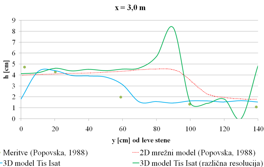
Slika 63: Prečni profil (od leve stene do sredine kanala) na razdalji 3 m od hipne razširitve; t = 10 s
