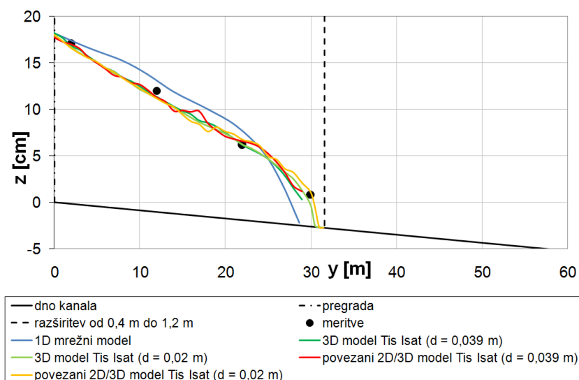
Slika 29: Primerjava med meritvami in rezultati simulacij 15,5 s po porušitvi pregrade – primer 1 (Džebo in sod., 2013 a)
