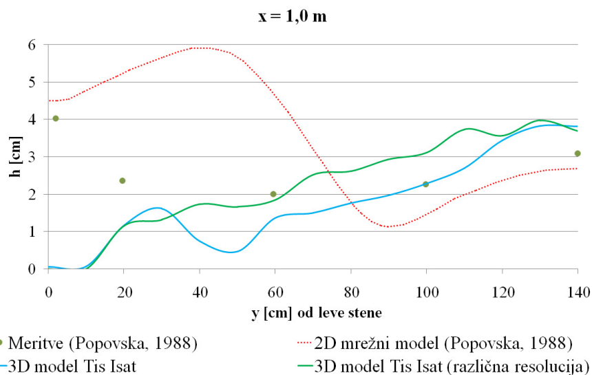
Slika 56: Prečni profil (od leve stene do sredine kanala) na razdalji 1 m od hipne razširitve; t = 7 \text{ s}
