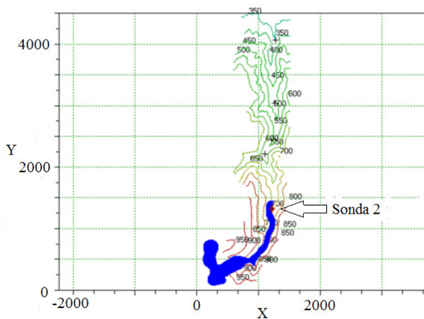
Slika 85: Tlorisni prikaz toka vode 62 s po poružitvi pregrade ( d = 2,5 m; bvis = 0,014 )
