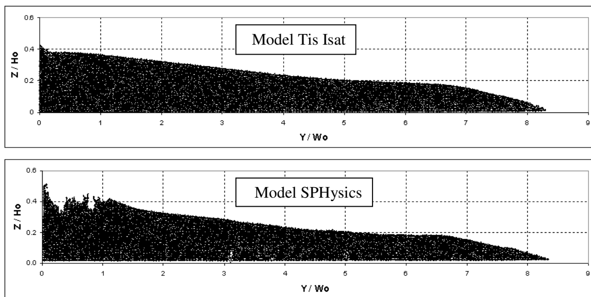
Slika 15: Primerjava napredovanja čela vala 0,3 s po porušitvi pregrade; H_o/W_o = 2 , število delcev je 50 x 100 (Petkovšek in sod., 2010 a)
