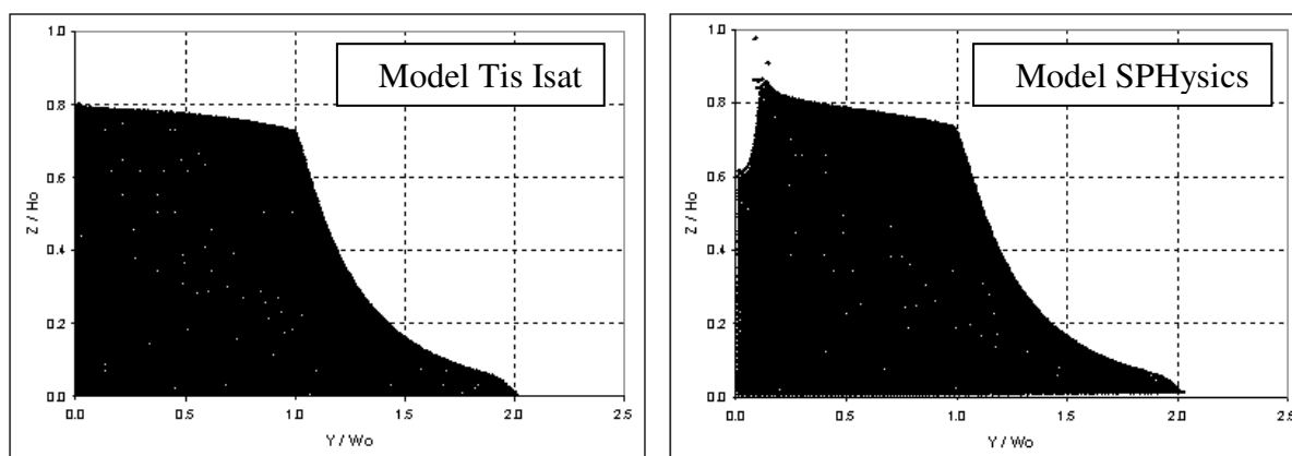
Slika 14: Primerjava napredovanja čela vala 0,08 s po poružitvi pregrade; H_o/W_o = 2 , število delcev je 50 x 100 (Petkovšek in sod., 2010 a)
