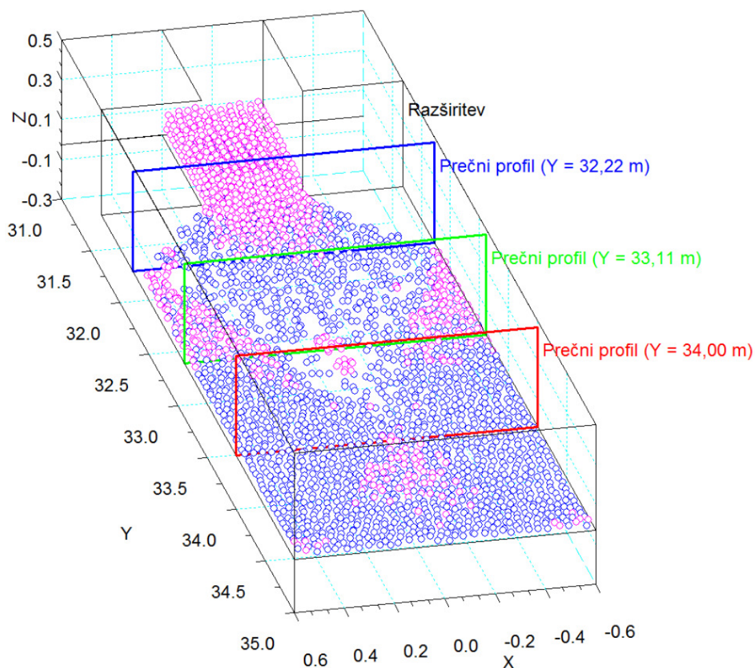
Slika 34: Aksonometrični pogled dela kanala z razširitvijo 45 s po porušitvi pregrade, simuliran z 3D modelom Tis Isat z večjimi delci. Delci v roza barvi prikazujejo območja z višjo, modri delci pa območja z nižjo globino (Džebo in sod., 2013 a)
