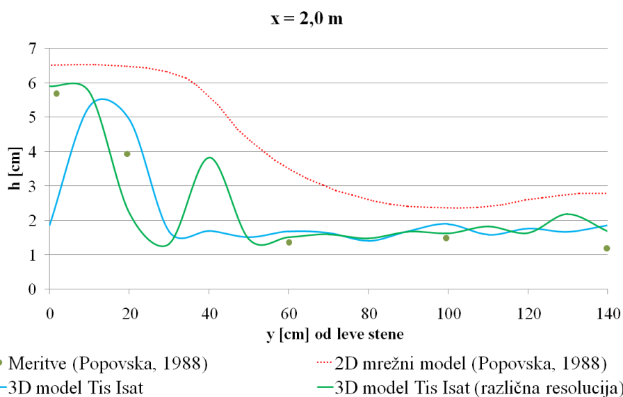
Slika 57: Prečni profil (od leve stene do sredine kanala) na razdalji 2 m od hipne razširitve; t = 7 \text{ s} .
