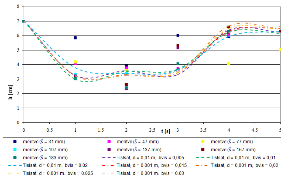
Slika 22: Višina vodnega stolpca v kanalu z zaporo (Džebo in sod., 2011)
