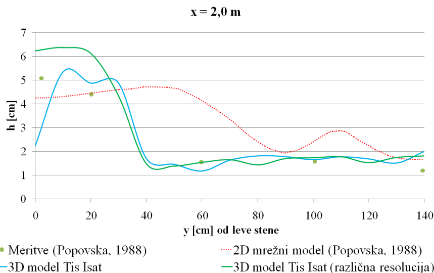
Slika 62: Prečni profil (od leve stene do sredine kanala) na razdalji 2 m od hipne razširitve; t = 10 s.
