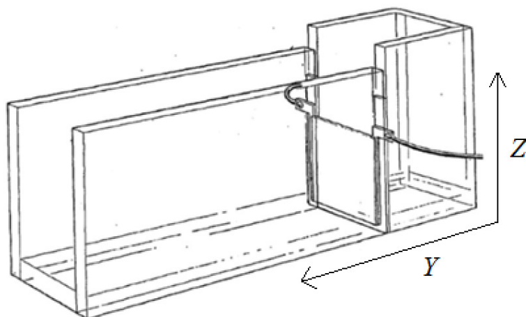
Slika 7: Fizični model (Martin in Moyce, 1952)
