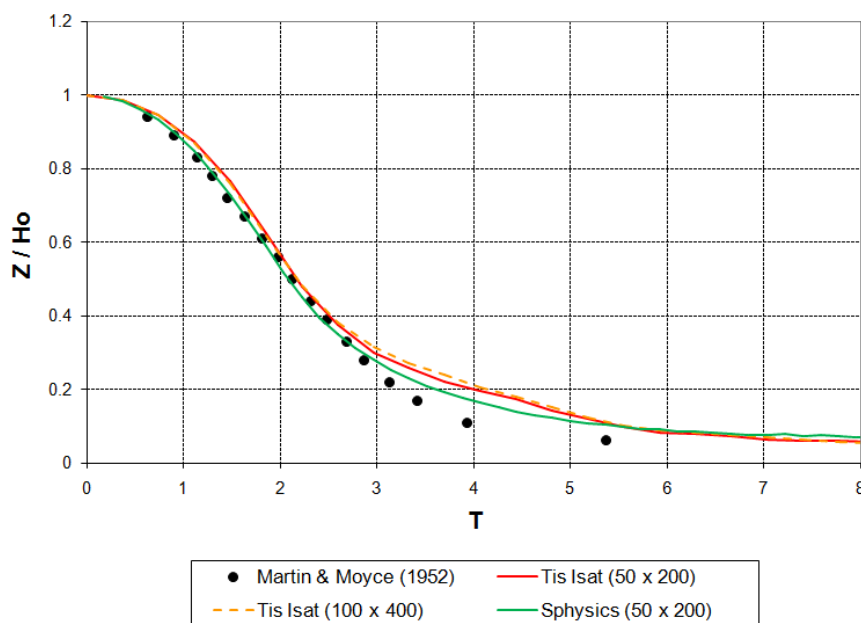
Slika 13: Relativna višina vodnega stolpca; H_o/W_o = 4 (Petkovšek in sod., 2010 a)
