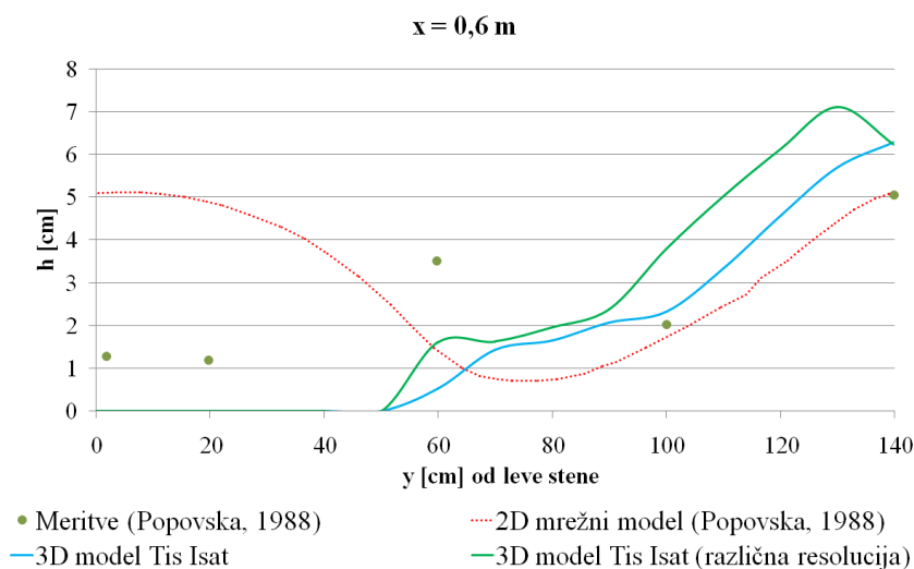
Slika 55: Prečni profil (od leve stene do sredine kanala) na razdalji 0,6 m od razširitve; t = 7 s.
