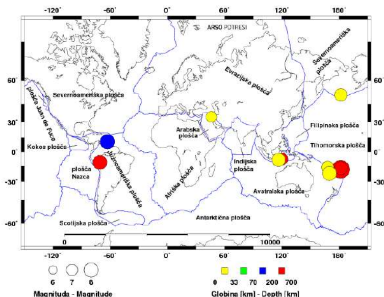
Slika 1. Najmočnejši svetovni potresi, avgust 2018
