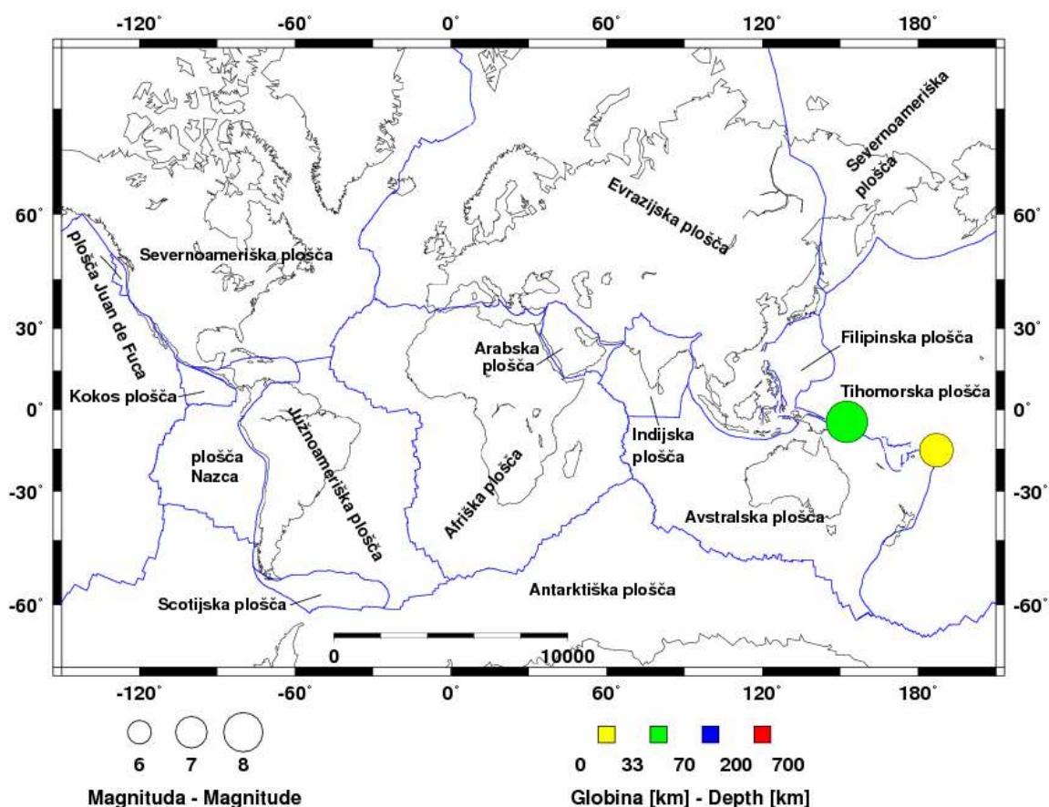
Slika 1. Najmočnejši svetovni potresi, marec 2015
