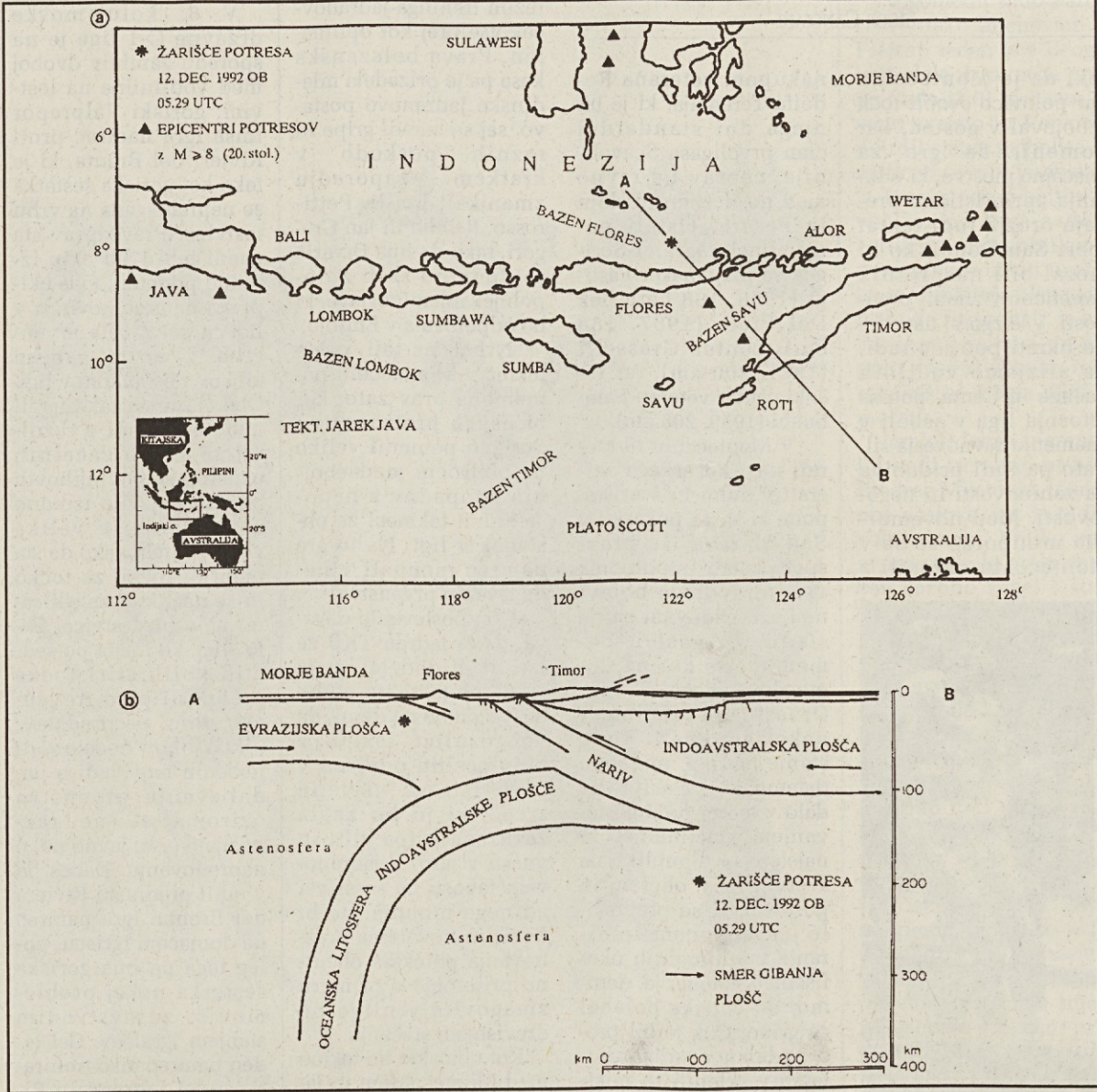
Geografska skica Indonezijskega arhipelaga in epicentri najmočnejših potresov v dvajsetem stoletju (2a). Geološki prerez ozemlja med bazenom Flores (morje Banda) na severozahodu in avstralskim šelfom na jugozahodu (2b).
