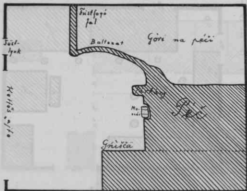
8. Prerez peči.
