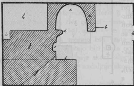
3. Prerez peči.
