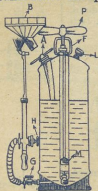
Prerez samodelne škopilnice.
