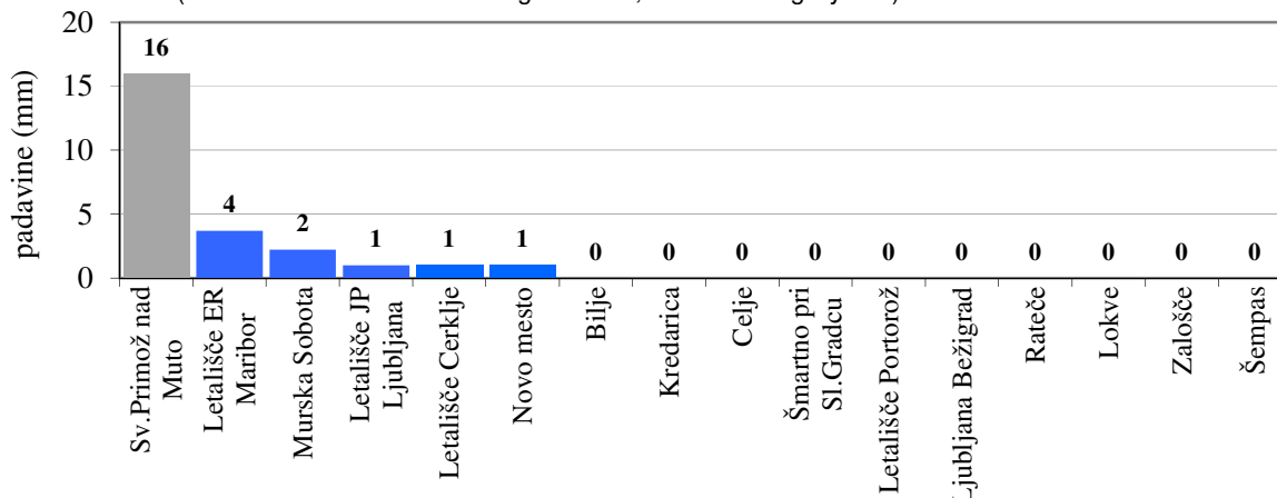
Slika 9. Višina padavin decembra 2016 na izbranih meteoroloških postajah po Sloveniji in na Lokvah
