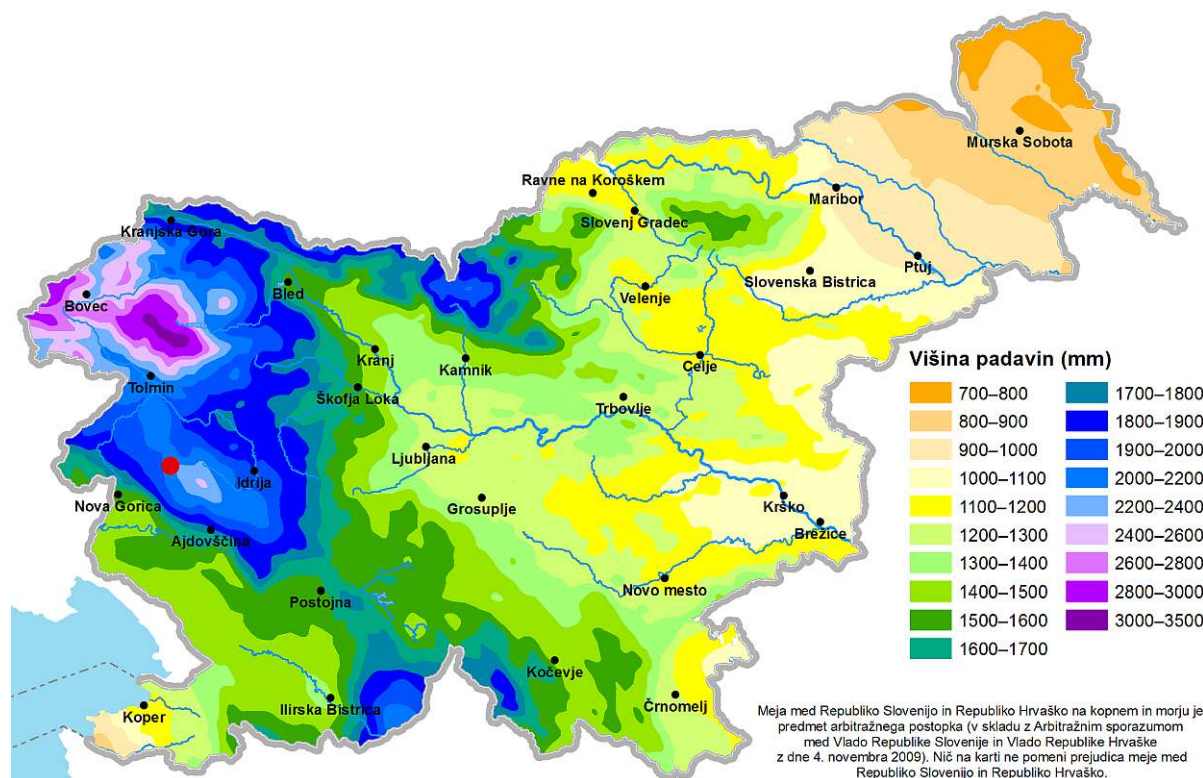
Slika 3. Letna povprečna višina padavin v Sloveniji, primerjalno obdobje 1981–2010. Lokacija postaje Lokve je označena rdeče
