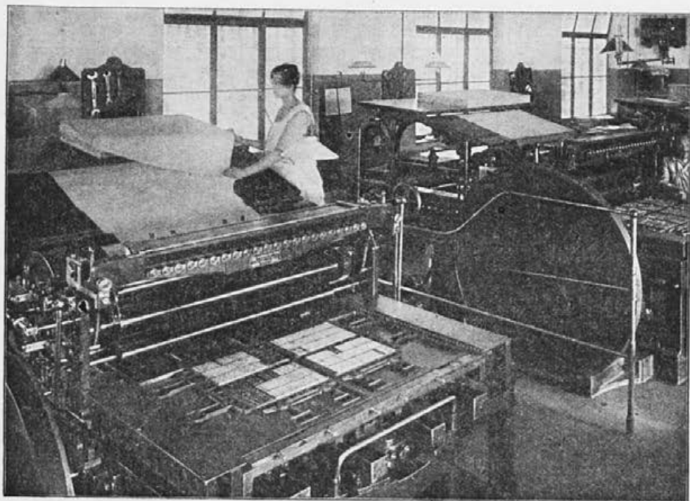
Tiskarski stroji „Učiteljske tiskarne“ v Ljubljani.
