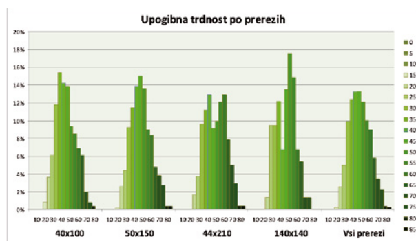
Slika 8. Porazdelitev upogibnih trdnosti po prerezi
