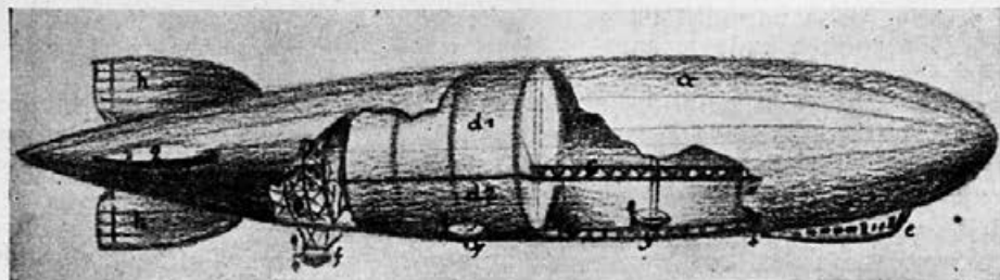
a = trupovo odevalo, b = ogrodje, c = srednji hodnik, d 1 = meh za nosilni plin, d 2 = meh za gonilni plin, e = glavni čolnič, f = strojnice, g = višinsko krmilje, h = smerno krmilje, i = glavni hodnik
