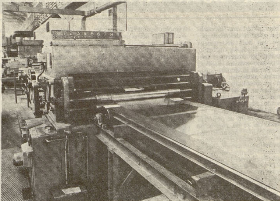
Rezanje pločevine
