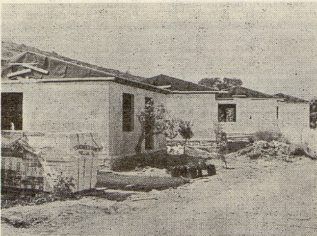
Izgradnja naših vikend hišic
