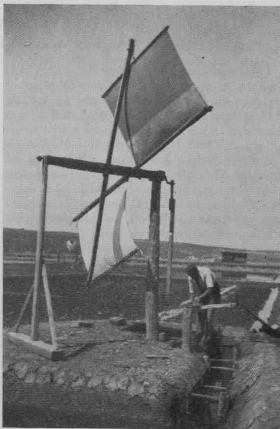
Vetrnica ali holandska črpalka na veter
