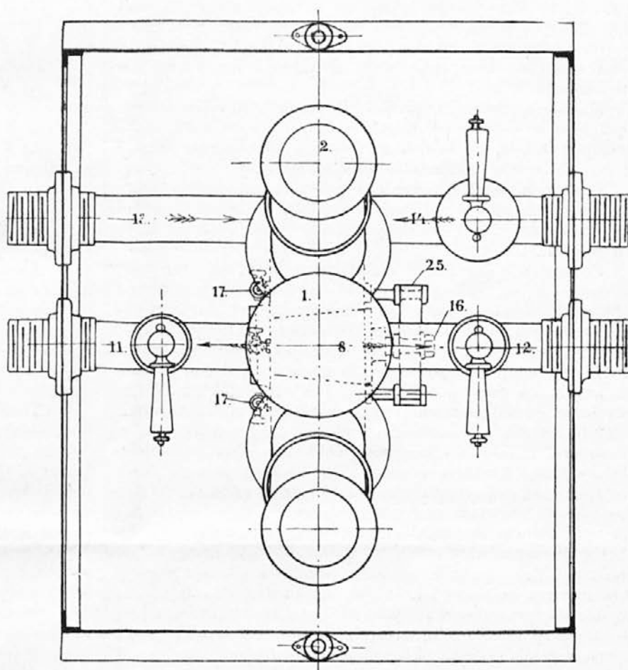
Temeljni načrt.
