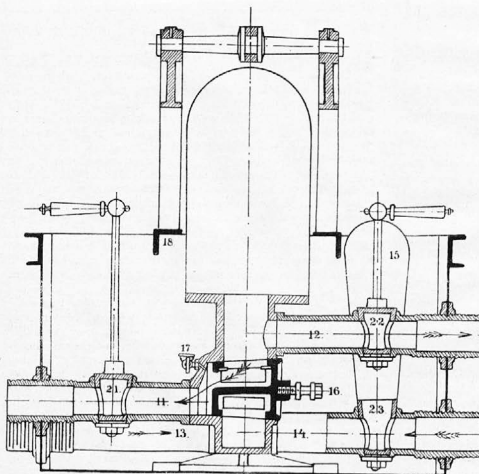
Poprečni rez.
