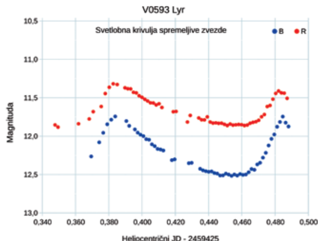
Slika 7: Rezultat meritev svetlobne krivulje pulzirajoče spremenljive zvezde V0593 Lyr. Spremenljivka je tipa delta Scuti, poimenovana tudi pritlikava kefeida. Periode pritlikavih kefeid so kratke, tipično nekaj ur, tako da lahko celotno krivuljo posnamemo v eni noči. Pri slikanju sta bila uporabljena modri filter B in rdeči filter R. Ustrezni krivulji sta prikazani na grafu. Zvezda radialno pulzira in posledično spreminja sij ter temperaturo, kar je tudi vidno iz razlike sija. Na osi X je datum v dnevih, na osi Y je navidezna magnituda. Zvezde kefeide so za astronome zelo pomembne, saj zanje velja zveza perioda-izsev, torej z meritvijo periode spremenljivke določimo izsev zvezde, to je absolutno magnitudo, in z meritvijo navideznega sija zvezde dobimo modul oddaljenosti, iz katerega potem izračunamo oddaljenost. S to metodo so izmerili oddaljenost kroglastih kopic in bližnjih galaksij, torej za razdalje, ki jih ne moremo izmeriti geometrijsko s paralakso. Meritve so bile opravljene na daljavo z robotskim teleskopom 29. 7. 2021 in obdelane s programom ASTAP [9], graf smo narisali v preglednici LibreOffice.
