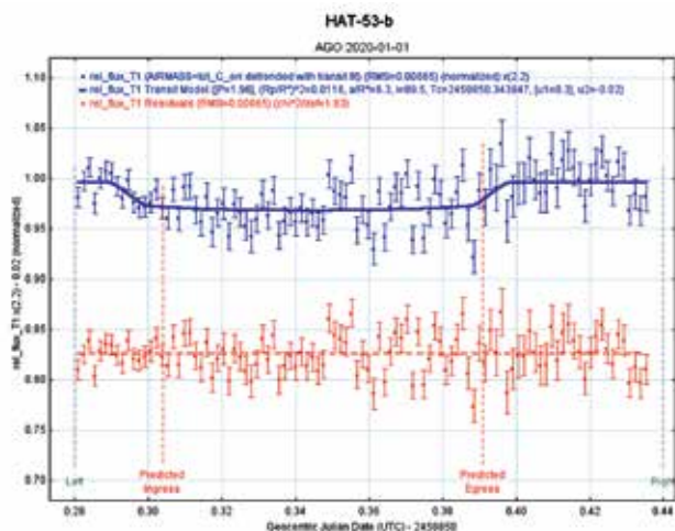
Slika 6: Mrk zvezde HAT-53, izmerjen ob prehodu planeta HAT-53- b. Modre točke so meritve sija iz slik, posnetih na daljavo z robotskim teleskopom 1. 1. 2020. Modra krivulja je model osončja HAT-53, rdeče točke prikazujejo ujemanje med modelom in meritvijo. Iz časa ponovitve sredine mrka določimo orbitalno periodo planeta, iz dolžine trajanja mrka kot naklona tirnice in iz globine mrka velikost planeta. Slike so bile obdelane s programom AstrolmageJ [8].
