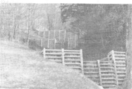
Lani je PUH obnovil pregrado v Petričevem grabnu. S tem je pripomogel k umiritvi tega hudournika ter zaščiti travnikov, polj in zgradb pred razdiralno močjo tega vodotoka (Foto: S. J.)
