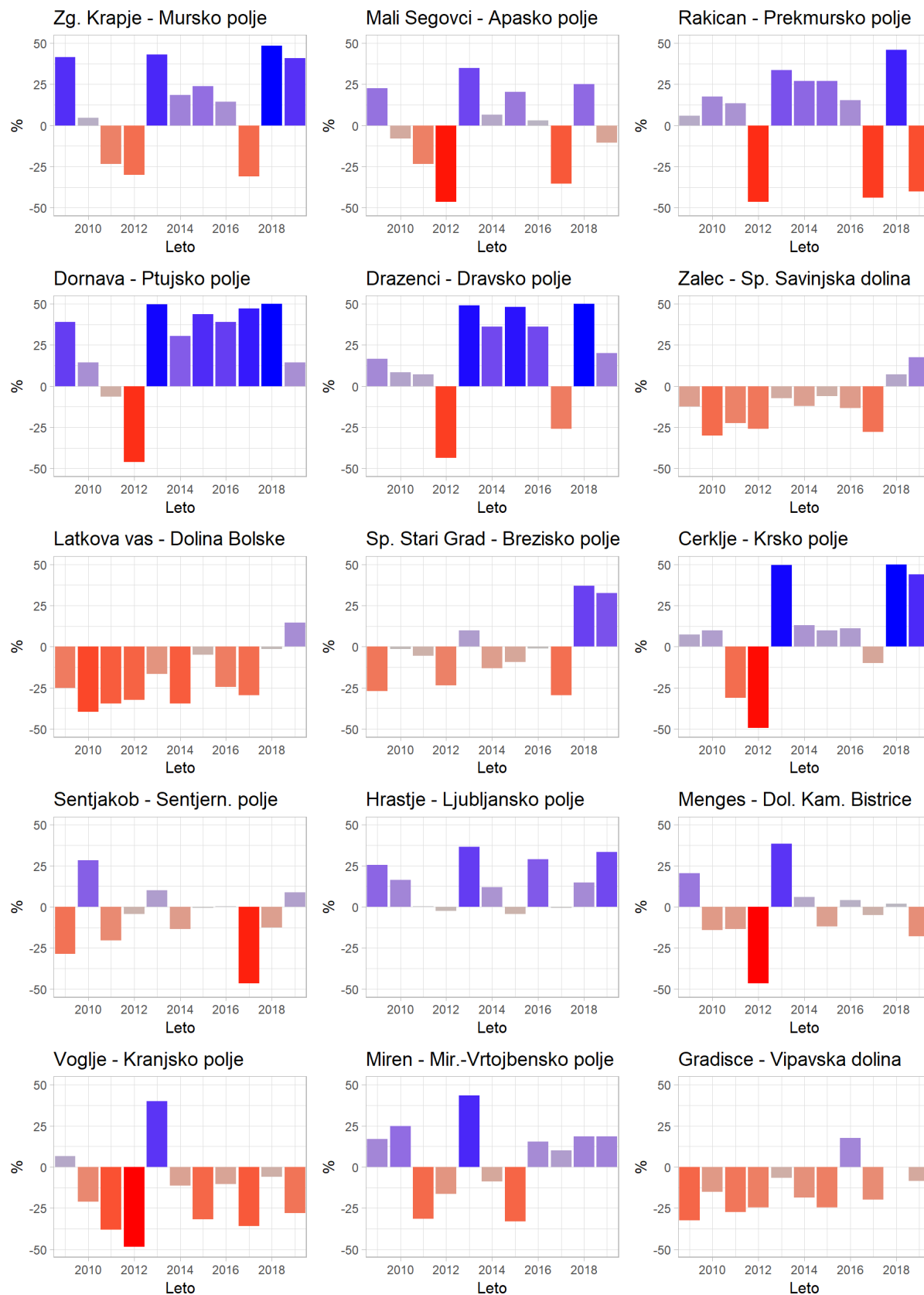
Slika 4. Odklon povprečne gladine podzemne vode junija 2019 od mediane dolgoletnih junijskih gladin v obdobju 1981–2010 izražene v percentilnih vrednostih
