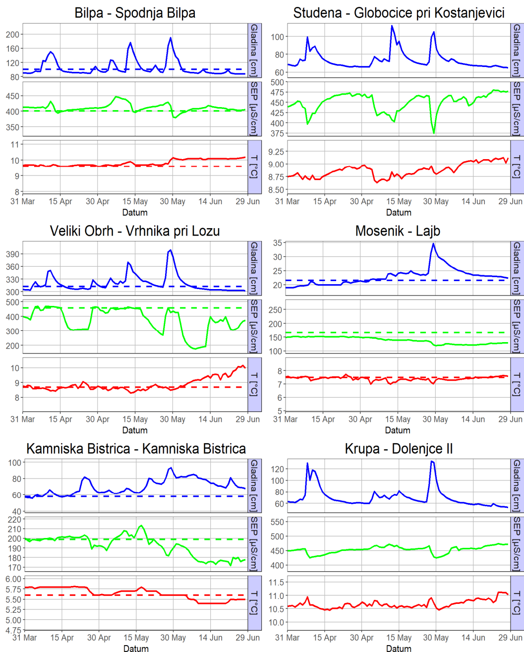
Slika 3. Nihanje vodne gladine (modro), temperature (rdeče) in specifične električne prevodnosti (zeleno) na izbranih merilnih mestih kraških izvirov med aprilom in junijem 2019
