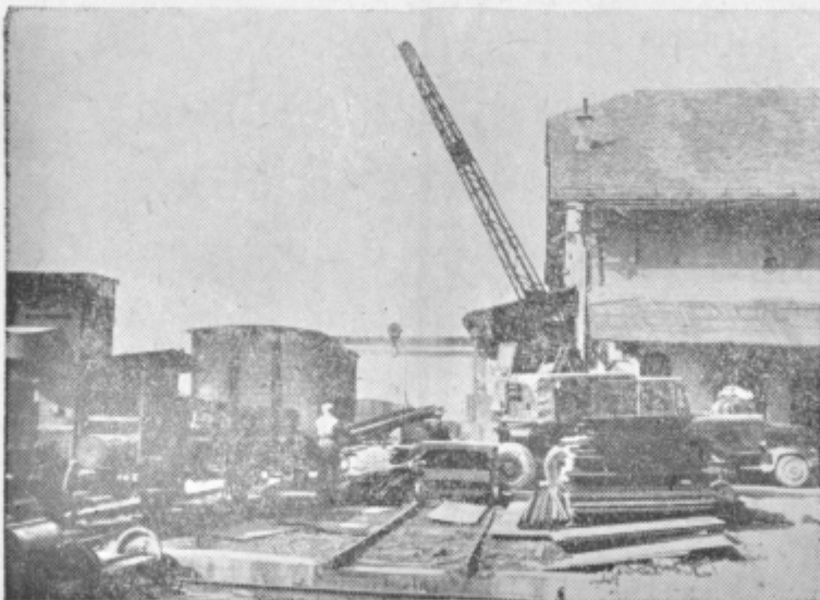
Motorno 5-tonsko dvigalo pri razkladanju železa
