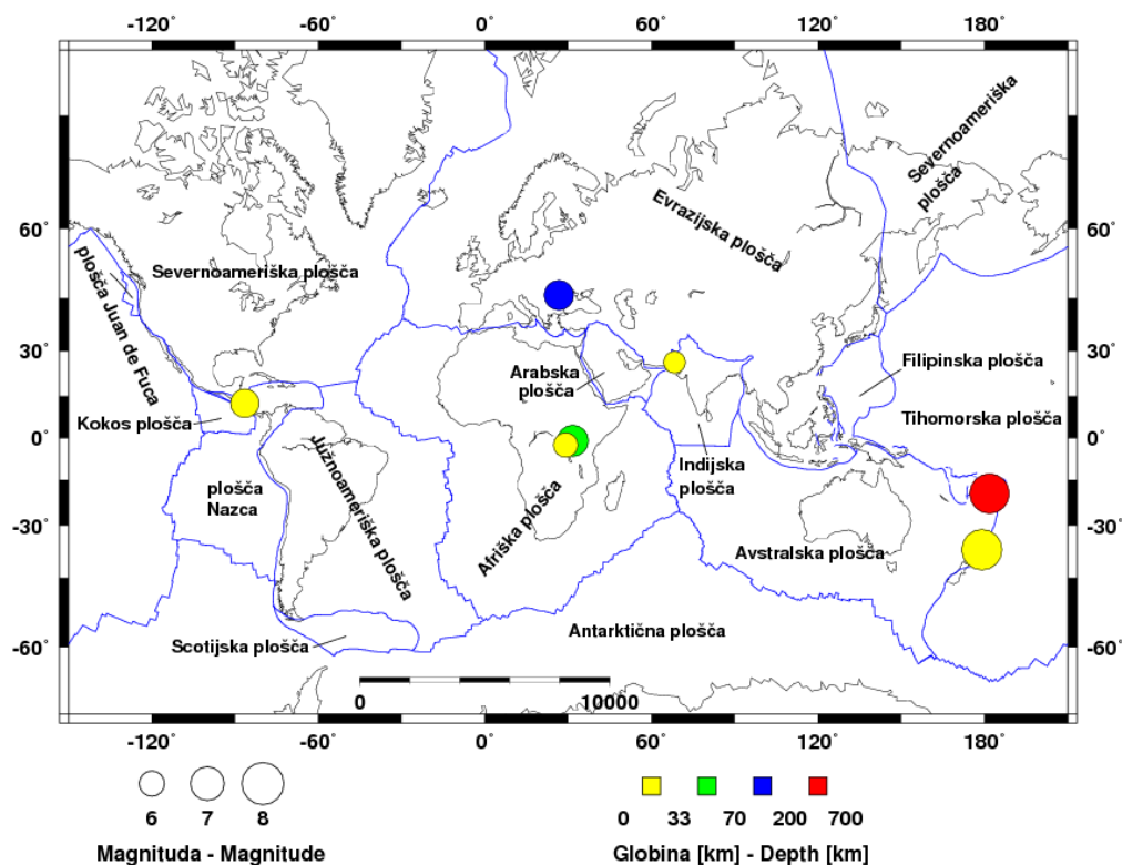
Slika 1. Najmočnejši svetovni potresi, september 2016
